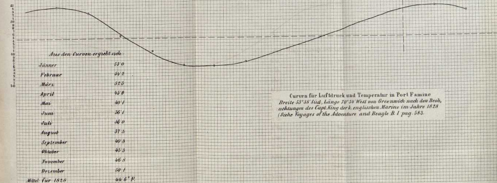
Thermometer Curve. Mittel derselben 44.6° F. für Mittag.
