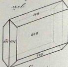
Cumarin.
