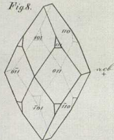
Citronensäure.
