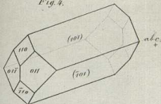
Hippuracresäure.
