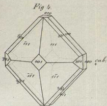
CaO, AcO 3 + 2(U 2 O 5 , AcO 3 ) + 2H 2 O.
