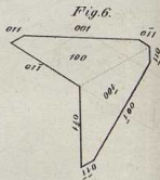
NaO, LiO, AcO 3 + 7H 2 O.
