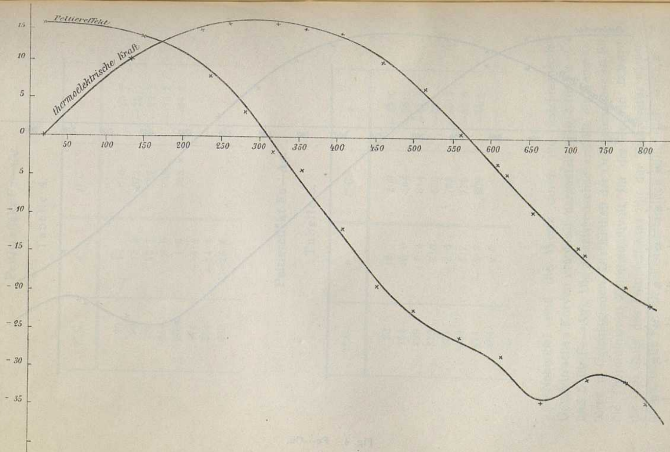
Fig. 5. Fe—Ag.
