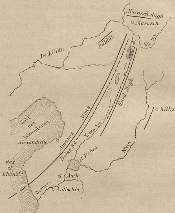
Fig. 5. Tektonische Skizze des nördlichsten Syrien.
