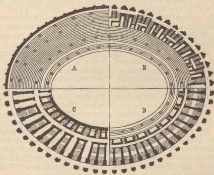
Grundriß des Amphitheaters zu Nîmes.
