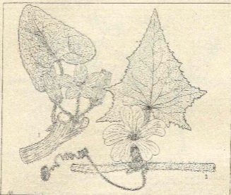
Pl. C. — 1. Eucalyptus Elaterium , portion de tige, 1/2 gr. n. — 2. Cucumis sativus , portion de tige, 1/2 gr. n.
