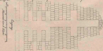
Grundriss des Ofens auf Scopelo.
