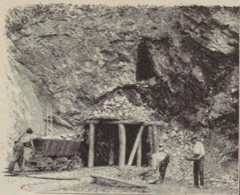
Schräm- oder Ritzstollen.
