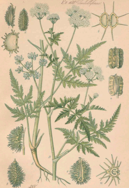
A. B. 1. 3. Torilis Anthriscus Smol. 4. 6. Lasopitium latifolium L. 7. 10. Targonia latifolia Hoffmann.
