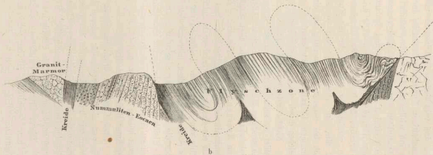
Die Entwicklung des Flysches und Alttertiärs bei Neubauern im Innthale. a Die natürlichen Aufschlüsse; b das aus den Aufschlüssen construirte Profil.
